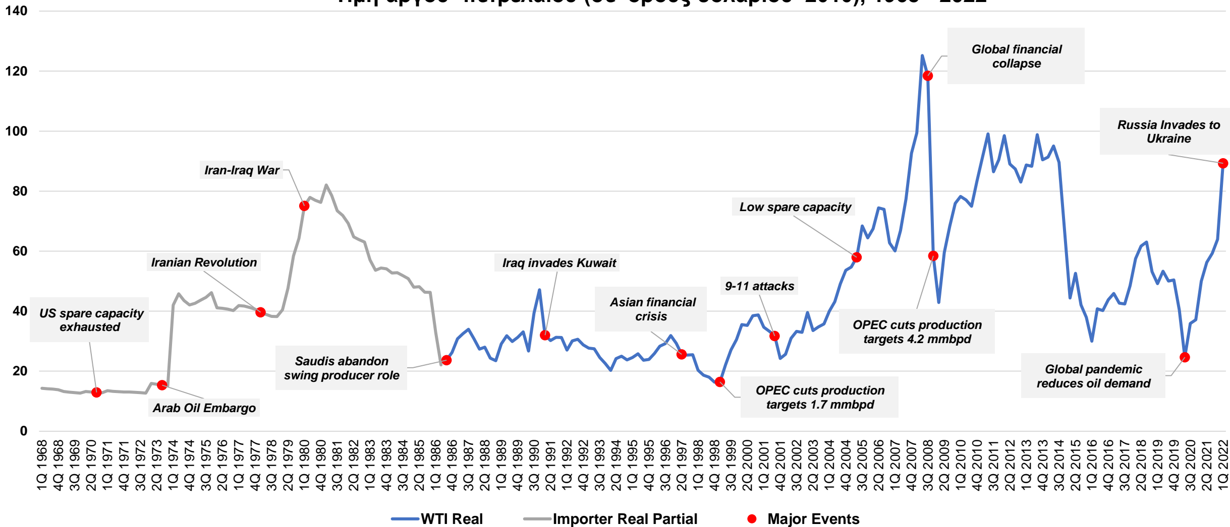
Τιμή αργού πετρελαίου (σε όρους δολαρίου 2010), 1968 - 2022
